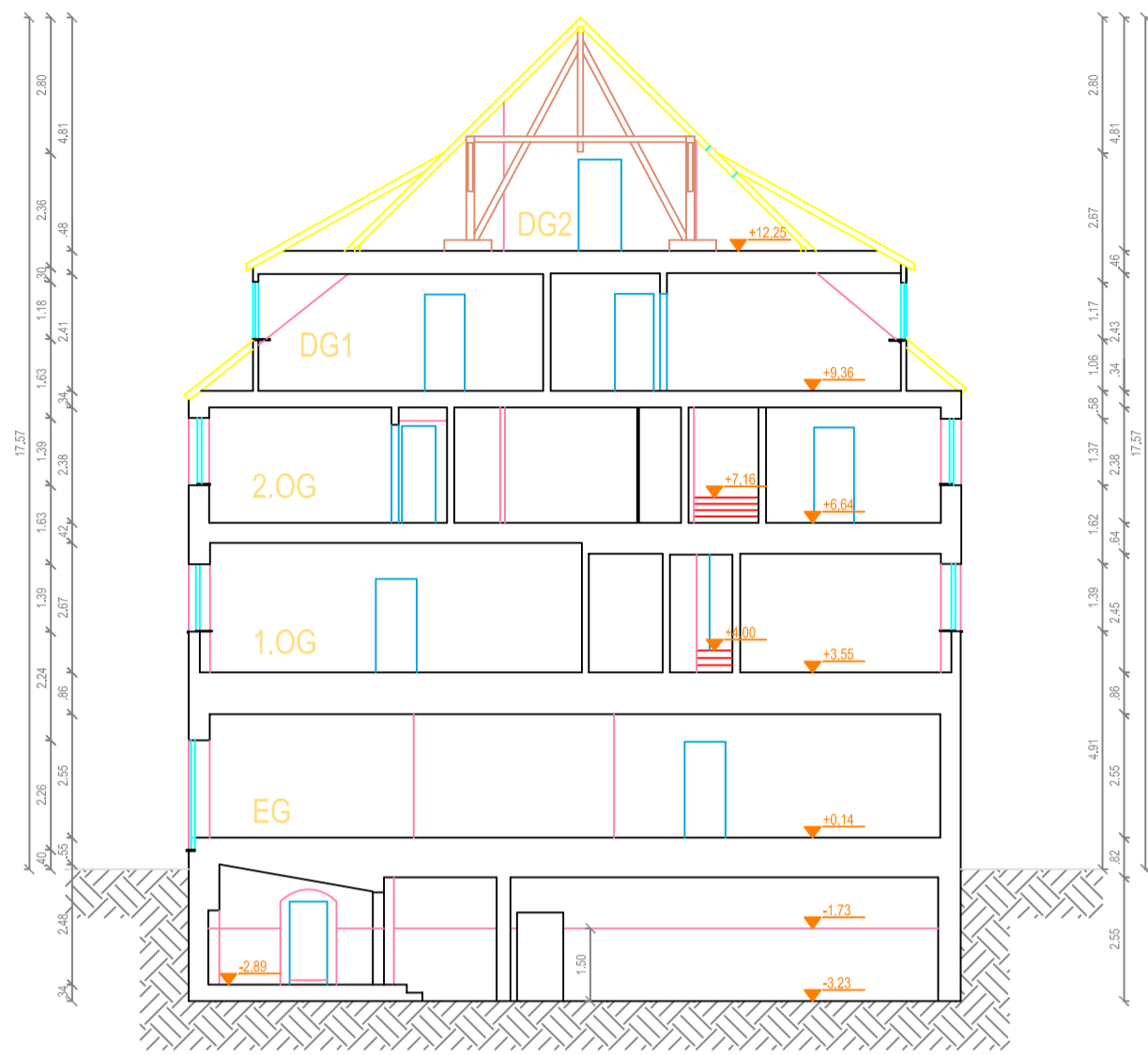
Schnitt C-C
