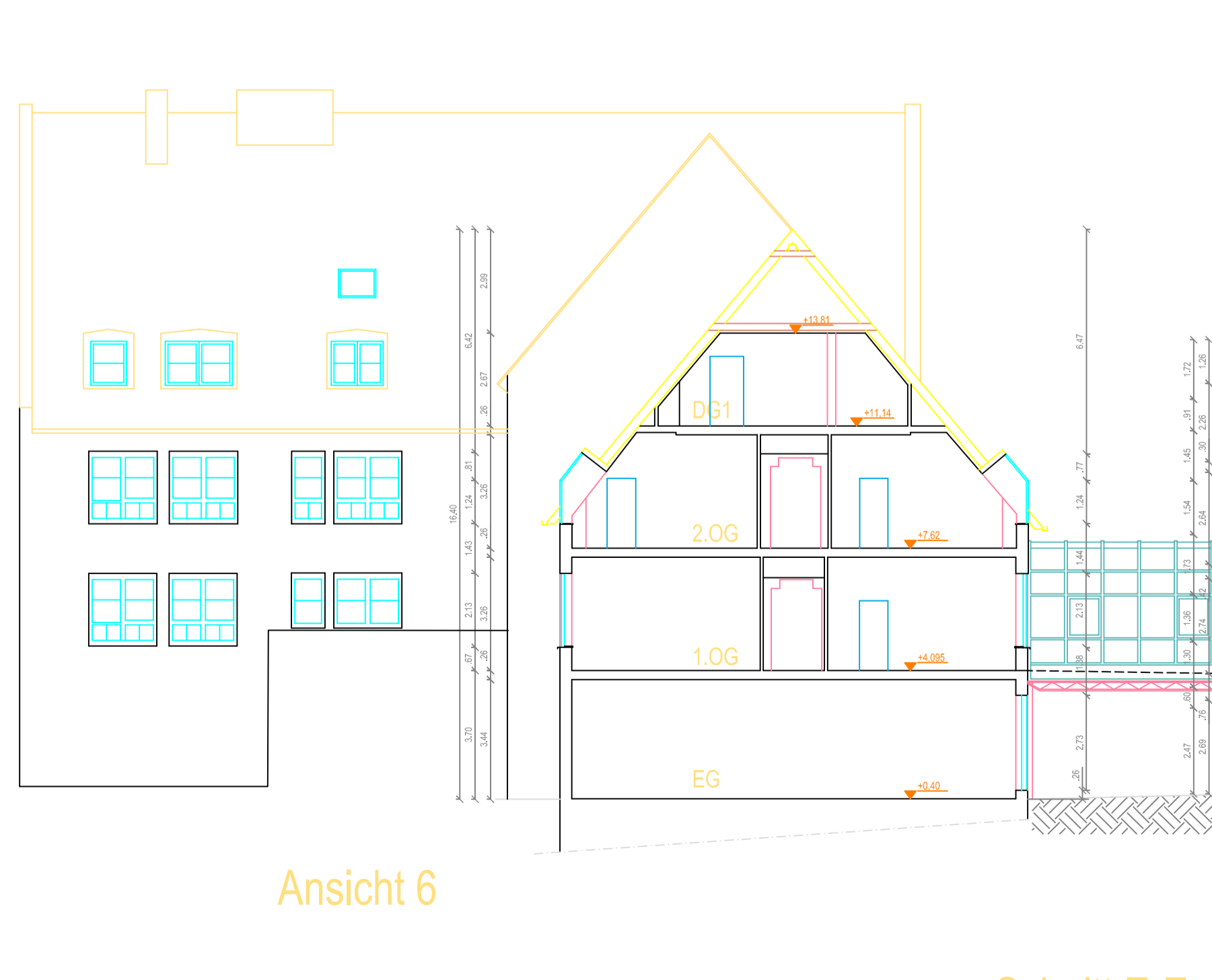
Schnitt E-E
